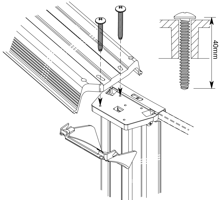
P.No.0345 5mmx40 Sheet Metal Screw
